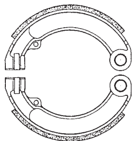
◀ cod. CP00211 Coppia ceppi \varnothing 125x19 Piaggio Vespa
