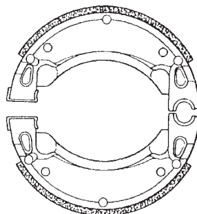
◀ cod. CP00239 Coppia ceppi \varnothing 110 x 25 MBK Booster 50 cc anteriore e posteriore
