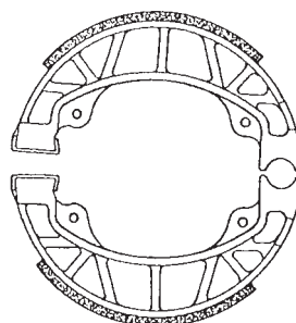
◀ cod. CP00240 Coppia ceppi \varnothing 110 x 25 Piaggio Skipper 50 cc posteriore
