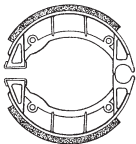
◀ cod. CP00200 Coppia ceppi \varnothing 90 x 18 con molle
