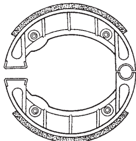
◀ cod. CP00201 Coppia ceppi \varnothing 105 x 20 con molle
